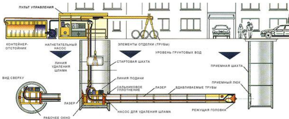
Рисунок 3. Схема микротоннелирования (4).
