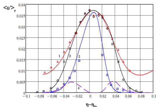
Рисунок 2: Профили условного и полного среднего безразмерной интенсивности пульсаций продольной скорости ASMTurb \langle u'_r \rangle = \langle u'^2_r \rangle_r / \Delta U^2 : 1- \Delta - \langle u'_r \rangle_t ; 2- \square - \langle u'_r \rangle_n ; 3- \circ - \langle u'_r \rangle = \langle u'^2 \rangle / \Delta U^2 ; 4- \langle u'^2 \rangle_{dop} / \Delta U^2 .
