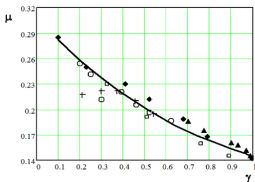
Рисунок 3: Распределения значений экспоненциального коэффициента Колмогорова \mu = \langle \mu \rangle_{iz} в зависимости от величины коэффициента внешней перемежаемости.
