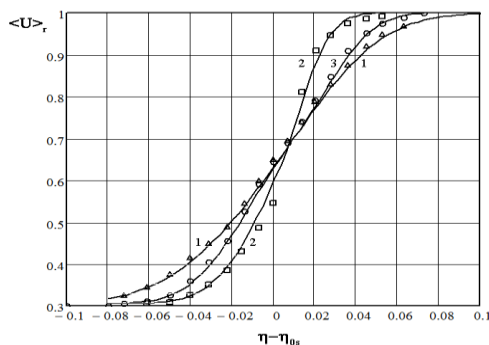
Рисунок 1: Профили условного и полного среднего безразмерной продольной скорости ASMTurb \langle U \rangle_r = \langle u \rangle_r / u_1 : 1– \Delta – \langle U \rangle_t ; 2– \square – \langle U \rangle_n ; 3– \circ – \langle U \rangle = \langle u \rangle / u_1 , u_1 и u_2 – скорости спутных потоков, u_2 / u_1 = 0.3 , \Delta U = u_2 - u_1 . Здесь и далее кривые линии – расчёт, значки – известные в литературе опытные данные.
