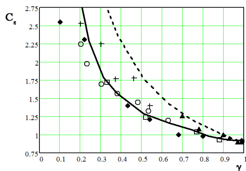
Рисунок 4: Распределения значений «второго» коэффициента Колмогорова C_\varepsilon = \langle C_\varepsilon \rangle_{iz} в зависимости от величины коэффициента внешней перемежаемости. Пунктирная кривая – расчет по модели [5], построенной в предположении локальной изотропии турбулентной жидкости.
