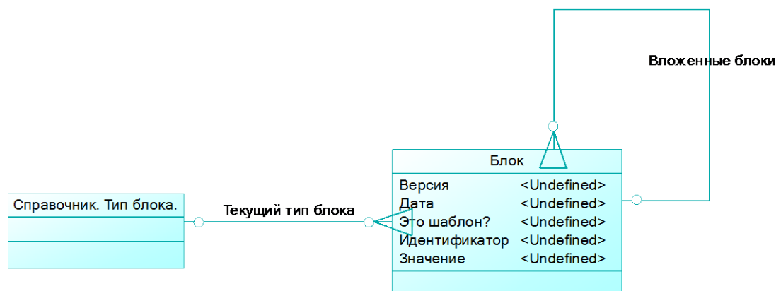
Рисунок 3 - схема данных
