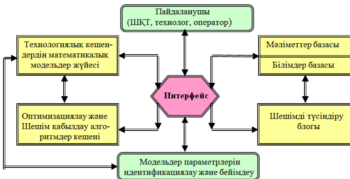
Сурет 1 - Мұнай өңдеу ы өндірісінің технологиялық кешендерін модельдеу және оптималды шешім қабылдау үшін ИШҚЖ құрылымы
