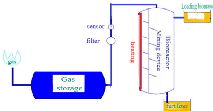
Сурет 2 - Биогаз қондырғысының сызбасы
