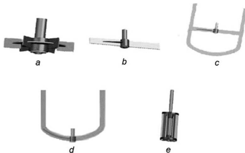
a - турбина; b - қалақша; c - жақтау; d - якорь; e - арнайы Сурет 1 - Механикалық араластыру құрылғылары
