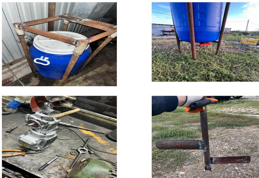
Сурет 2 - Биогаз қондырғысы
