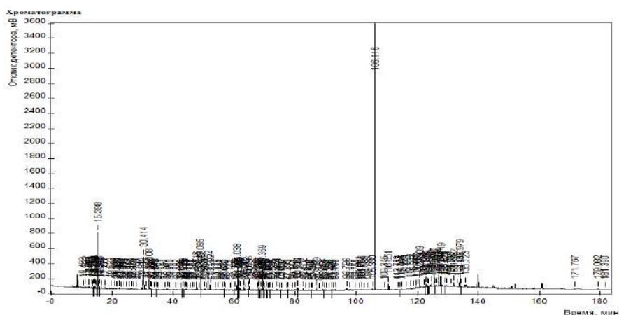
Сурет 2 Тоқыма сымы карбонизациясы мен активациясы нәтижесінде алынған сұйық өнімдердің хроматограммасы
