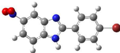
Рисунок 2 2(-4-бромфенил)-5-нитро-1Н-бензимидазол ( C_{13}H_9N_3O_2Br )
