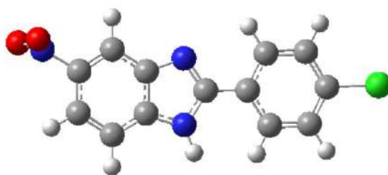
Рисунок 1 2(-4-хлорофенил)-5-нитро-1H-бензимидазол (C 13 H 9 N 3 O 2 Cl)
