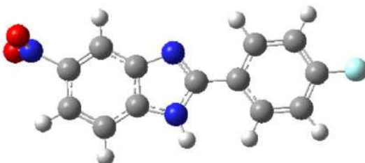
Сурет 3 2(-4-фторфенил)-5-нитро-1Н-бензимидазол ( C_{13}H_9N_3O_2F )
