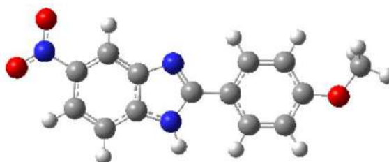
Сурет 4 2-(4-метокси)-5-нитро-1Н-бензимидазол ( C_{14}H_{11}N_3O_3 )
