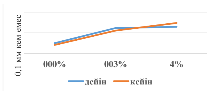
Сурет 2 БПБ қоспасының тотығуға дейінгі және кейінгі иненің ену тереңдігі
