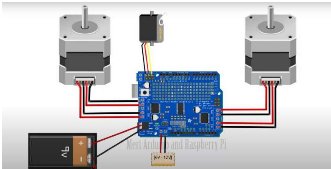
1 сурет. Жобаның сызбалық схемасы
