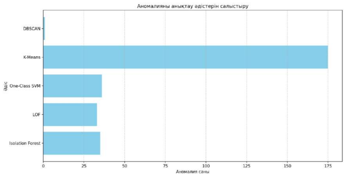
Сурет 1. Аномалияны анықтау әдістерін салыстыру
