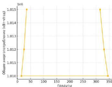
Рисунок 2. Ориентация в зависимости от общей энергии на объекте в год
