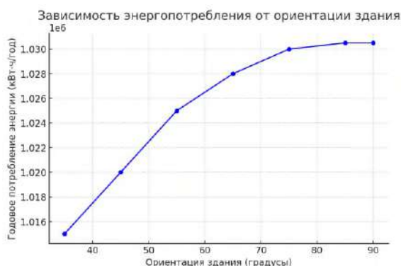
Рисунок 1 - Ориентация в зависимости от общей энергии на объекте в год
