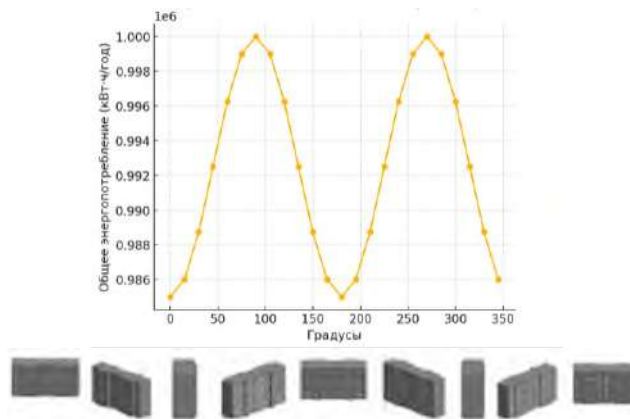
Рисунок 3. Ориентация в зависимости от общей энергии на объекте в год
