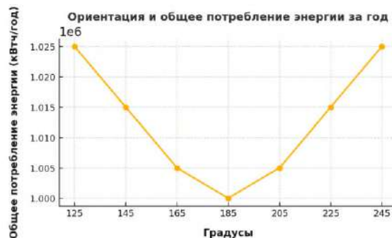
Рисунок 4. Ориентация в зависимости от общей энергии на объекте в год
