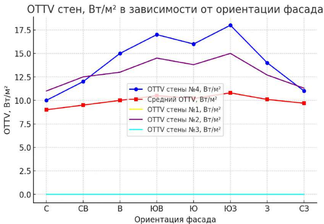
Рисунок 5. Результаты расчетов ОТТВ
