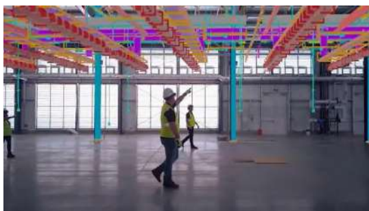
Рис.5. Визуализация инженерных сетей здания на площадке, при помощи технологии дополненной реальности
