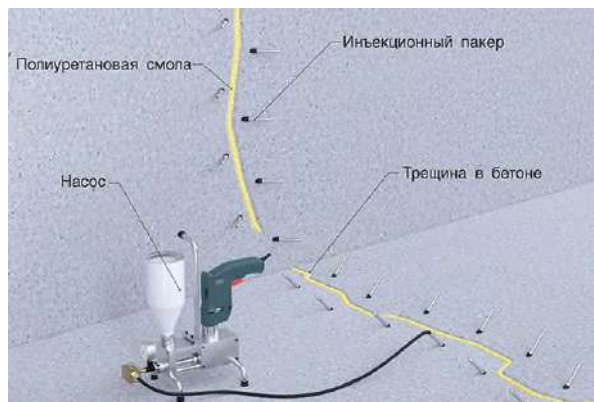
Рис.6 схема инъектирования бетона
