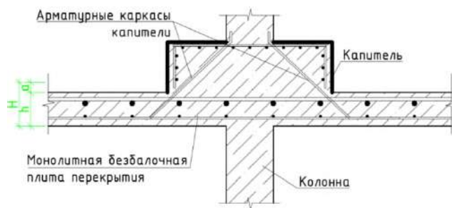
Рисунок 2. Повышение несущей способности посредством использования капители, расположенной на перекрытии
