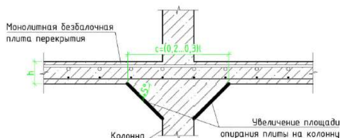
Рисунок 1. Повышение несущей способности посредством увеличения зоны опирания
