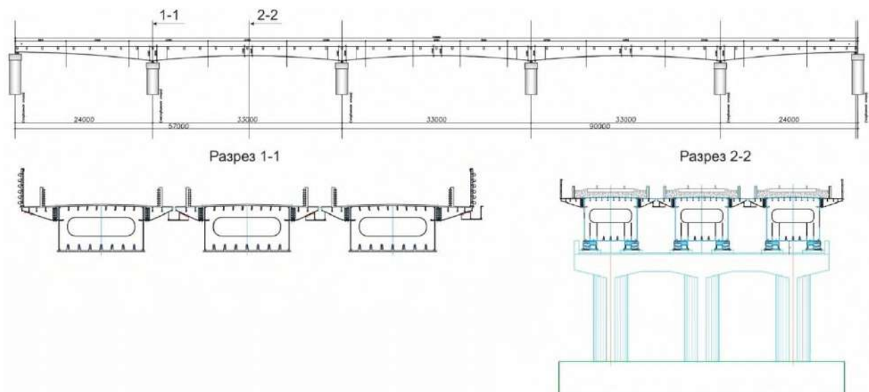
Рисунок 2. Металлические балки
