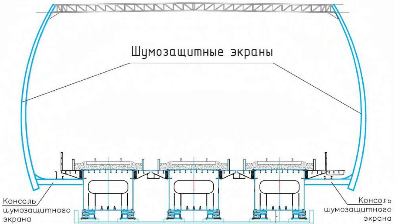
Рисунок 2. Шумозащитный экран.
