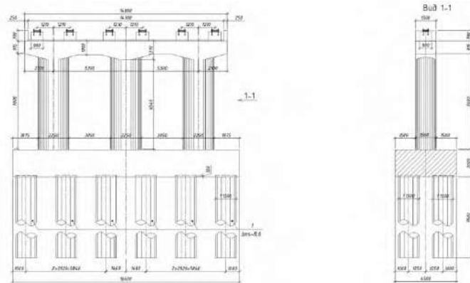
Нагрузки: собственный вес, подвижной состав, торможение, центробежные силы; Рисунок 1. Железобетонные опоры
