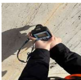
Рис.7, 8 Определение прочности бетона в конструкции ультразвуковым методом и методом ударного импульса
