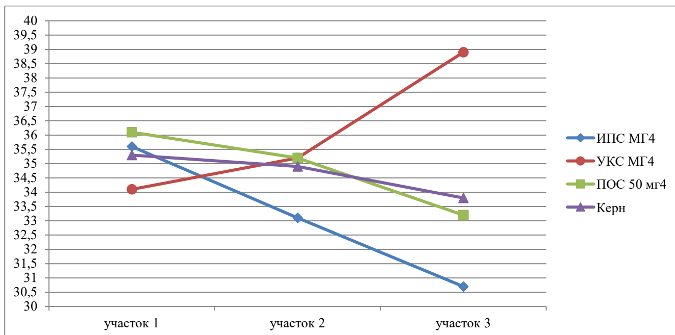
Рис.6 Диаграмма сравнения результатов исследования прочности бетона
