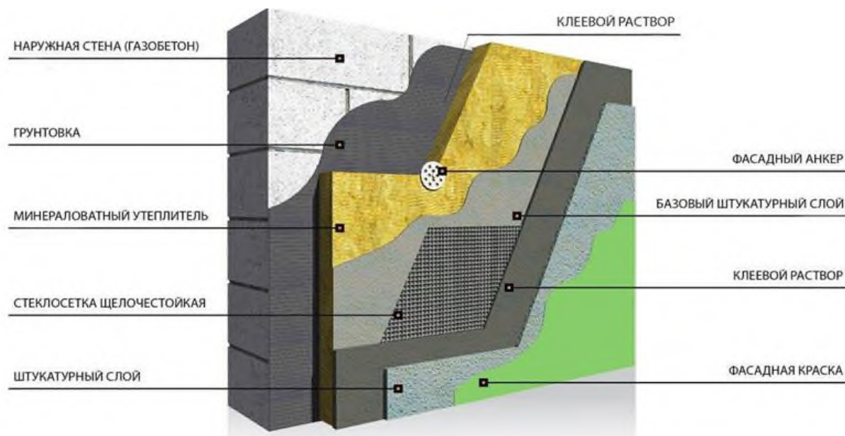
Рис.1 – Состав фасадного слоя
