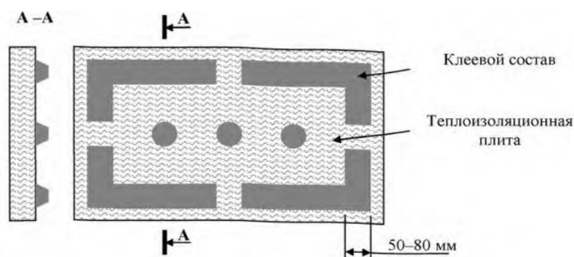
Рис.2 Схема примера нанесения клеевого состава на теплоизоляционную плиту
