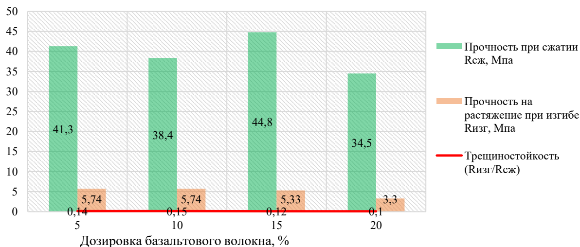
Рис.2. Результаты исследования оптимальной дозировки базальтового волокна [5]
