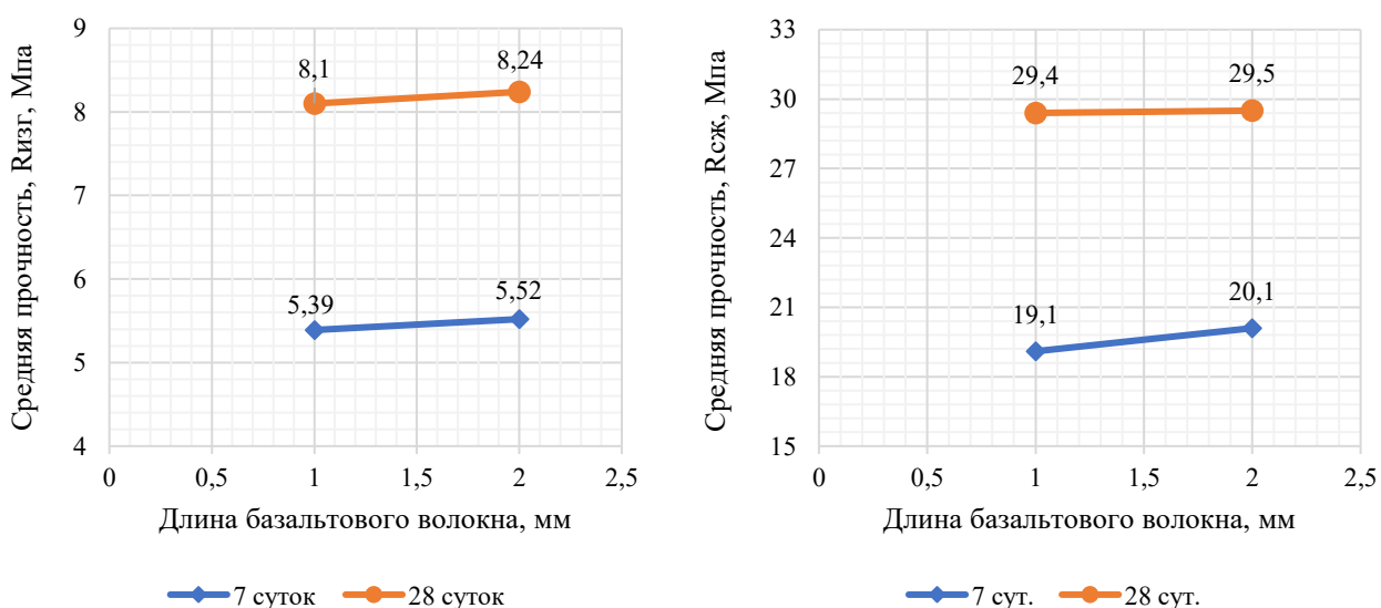
Рис.3. Прочностные характеристики мелкозернистого бетона, армированного с различным процентным содержанием рубленого волокна и добавлением пластификатора СП-3 [4]
