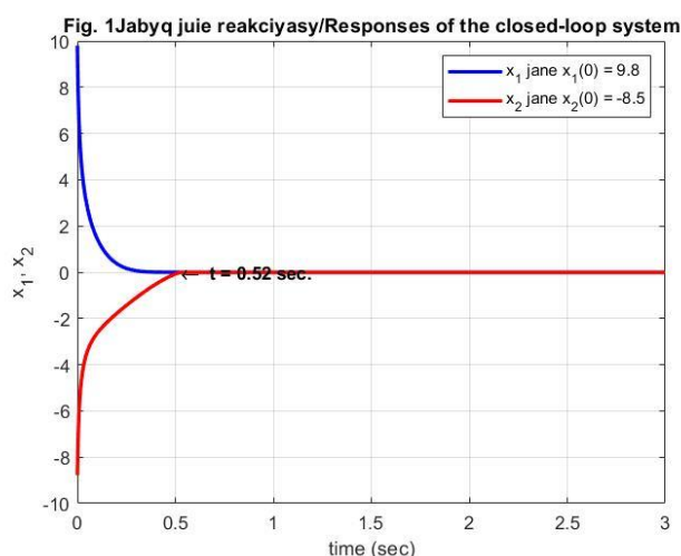
1-сурет. Жабьқ жүйе реакциясы ( t=0.52c )
