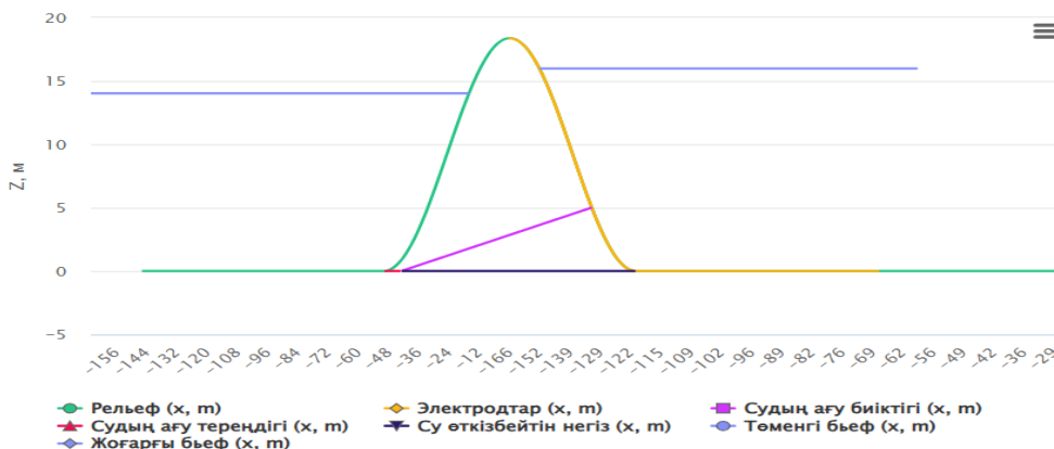
Сурет 1 Платформадағы су өткізбейтін негізі және утечкасы бар дамба және жоғарғы-төменгі бьеф геометриясы
