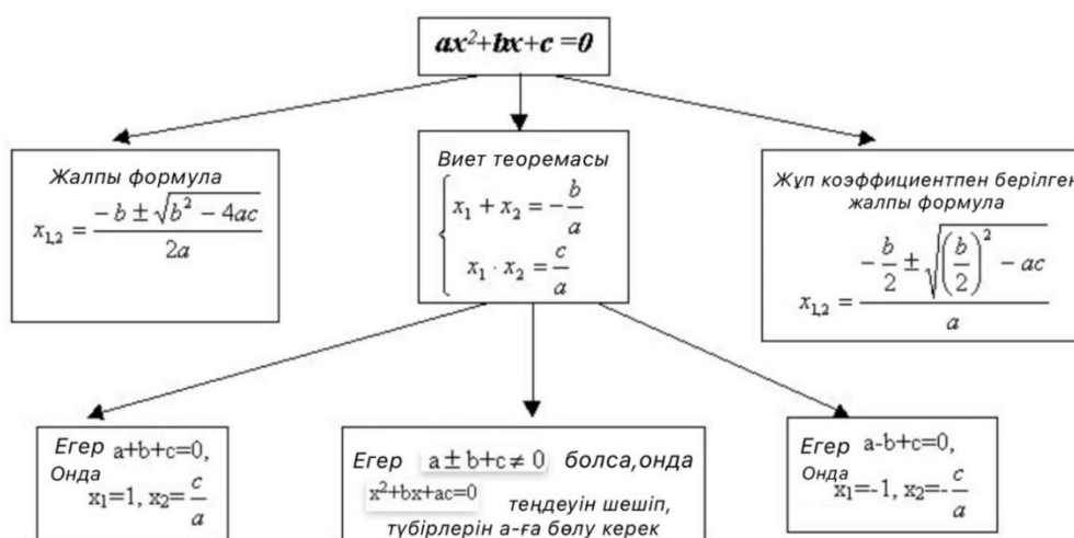
Сурет 3. Толық квадраттық теңдеулерді шешу әдістері
