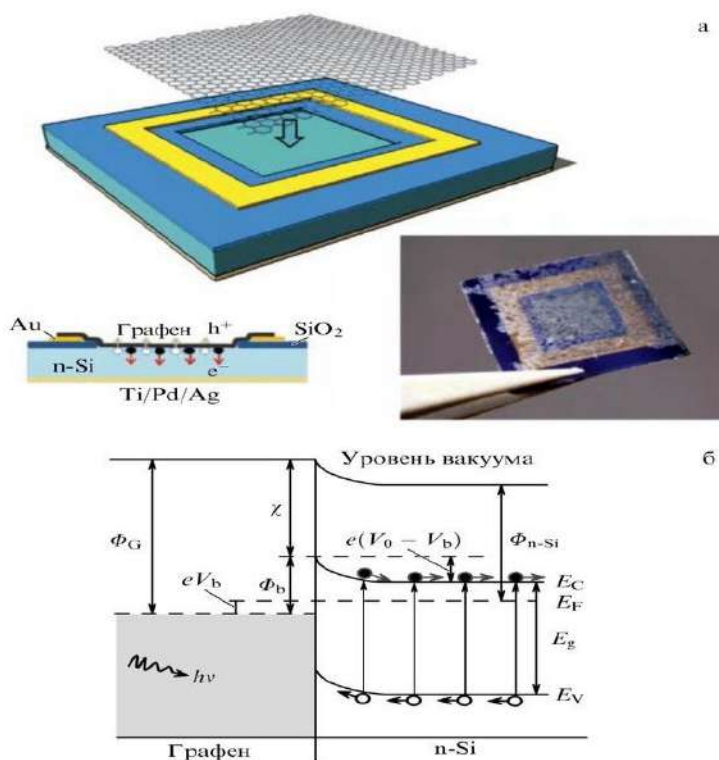
Сурет 1. Эксперименттік үлгінің схемалық көрінісі және суреті.
