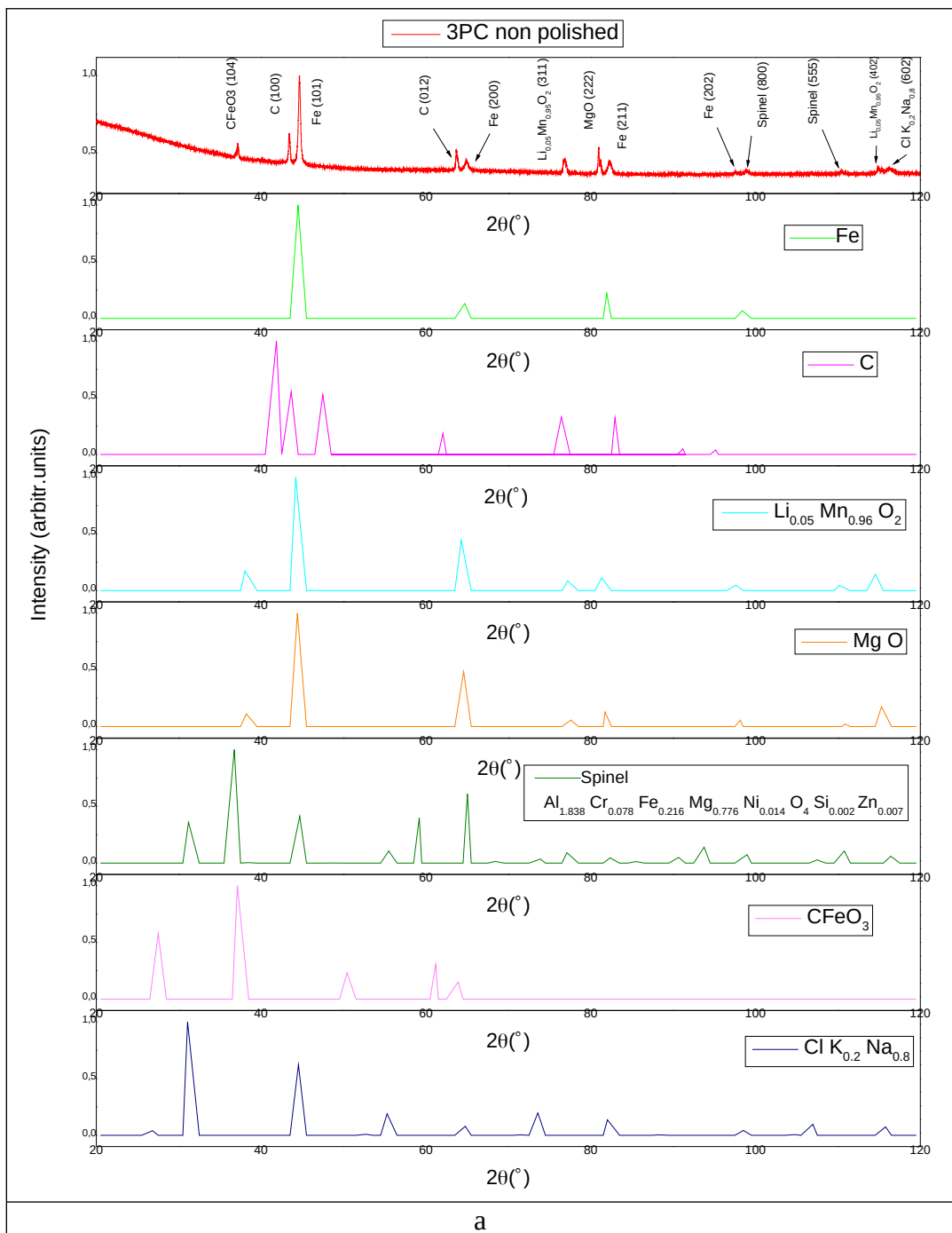
Рис.3 - РФА стали Зпс: (а)- исходного образца, (б)-шлифованного образца
