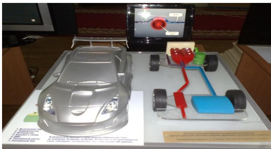
Рисунок 1 – Модель автомобиля с системой питания на крекинг-газе
