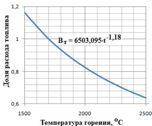
Рисунок 2 – Зависимость доли расхода топлива от температуры горения
