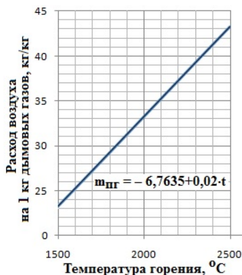
Рисунок 1 – Зависимость расчётного расхода воздуха от температуры горения
