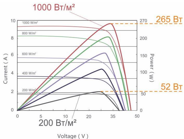
Рисунок 5. График зависимости мощности солнечной панели от освещенности [7].
