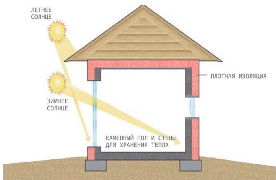
Рисунок 1. Устройство пассивной солнечной энергетической системы [3].
