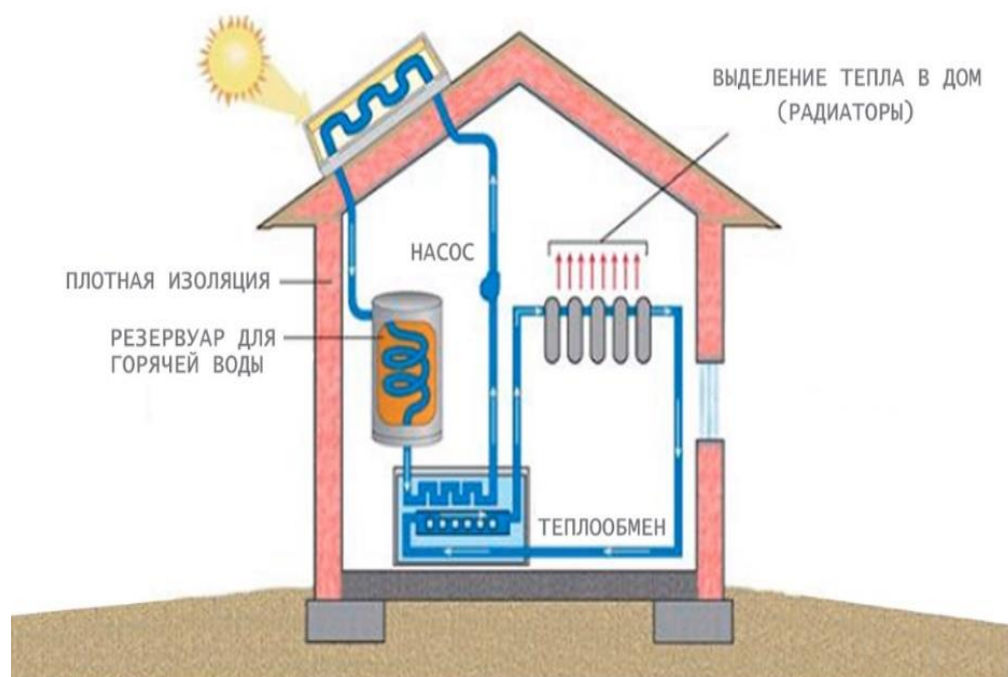
Рисунок 2. Устройство активной солнечной водонагревательной энергетической системы [3].
