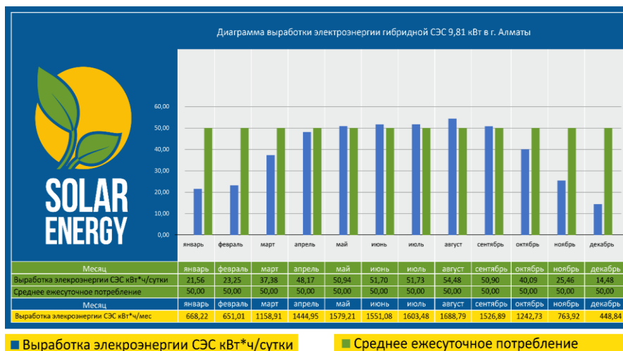
Рисунок 6. Диаграмма выработки электроэнергии гибридной СЭС 9,81 кВт*ч в г. Алматы [8].
