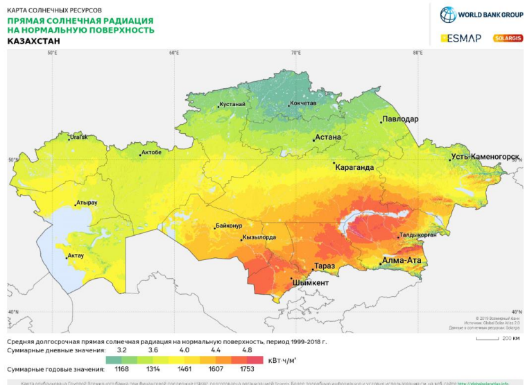
Рисунок 3. Прямая солнечная радиация на нормальную вертикальную или горизонтальную поверхность [6].
