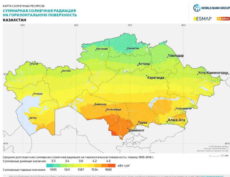
Рисунок 4. Суммарная солнечная радиация на горизонтальную поверхность [6].
