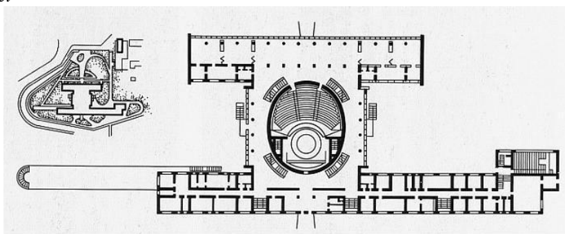
6-сурет. Н. Островский атындағы бұрынғы Пионерлер мен оқушылар сарайы, 1962-1965 жж., Киев қаласы
