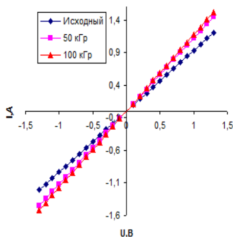
Рисунок 1. Вольтамперных характеристики исследуемых Со-НТ
