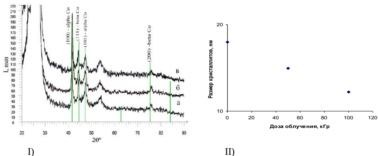
Рисунок 3. I) Рентгеновские дифрактограммы Co НТ; II) График зависимости размеров кристаллитов от дозы облучения. Буквами а,б,в на дифрактограммах обозначены дозы облучения а) исходный, б) 50 кГр, в) 100 кГр.
