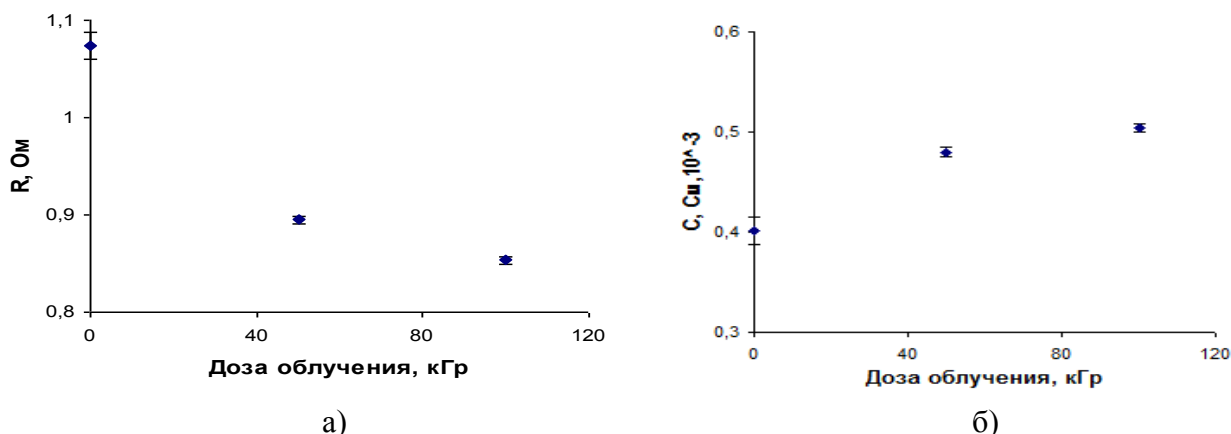
Рисунок 2. а) График зависимости изменения сопротивления от дозы облучения; б) График зависимости изменения проводимости от дозы облучения Co – НТ
