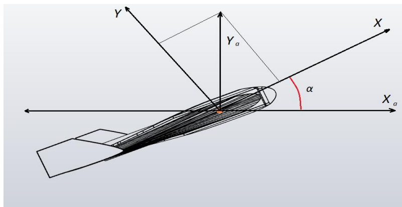
Рисунок 1 - Подъемная сила и лобовое сопротивление от угла атаки в системе координат
