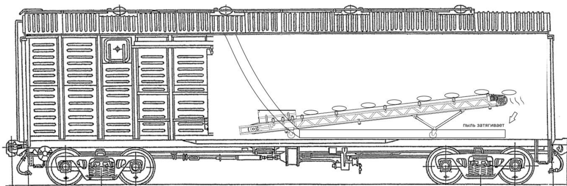
Рисунок 1 - Схематический набросок модели осуществления погрузки мешкотары с пылящим характером груза в крытом товарном вагоне с использованием ленточного конвейера
