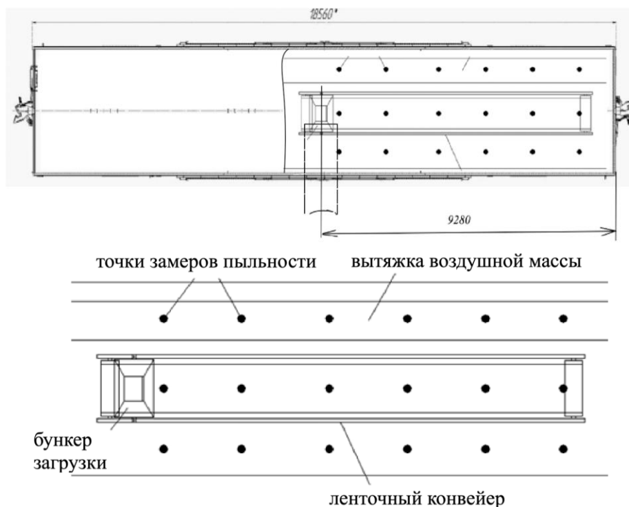
Рисунок 4 - Расположение точек измерения концентрации пыли
