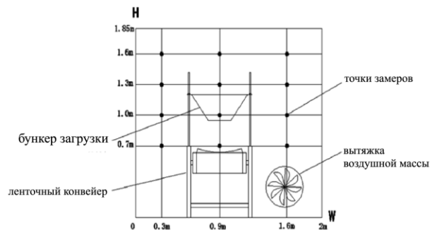
Рисунок 3 - Расположение точек замеров пыльности
