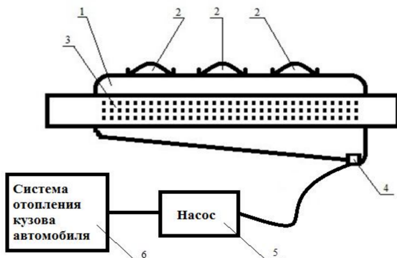
1 – корпус; 2 – ультразвуковые устройства; 3 – отверстия; 4 – краник; для слива образовавшейся смеси; 5 – насос; 6 – система отопления кузова автомобиля
