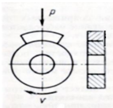
Рисунок 1 - Схема испытания на изнашивание цилиндрического колесного ролика и рельсового вкладыша ( P=73,5 МПа, V=36 м/мин)
