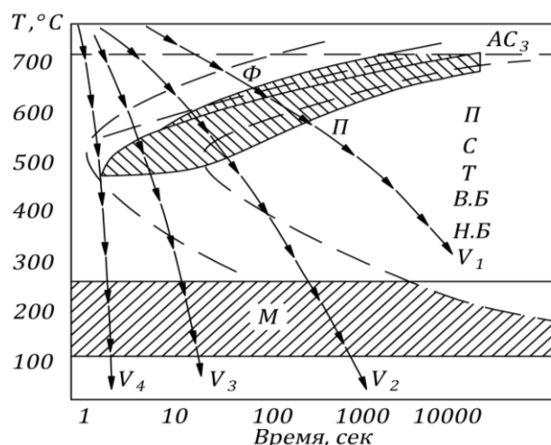
Рисунок 4- Неоднородная градиентно-слоистая структура поверхностной зоны плазменно-закаленной стали
