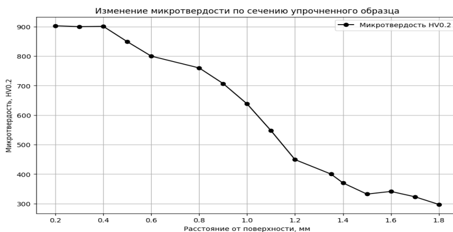
Рисунок 3- Изменение микротвердости по сечению упрочненного образца
