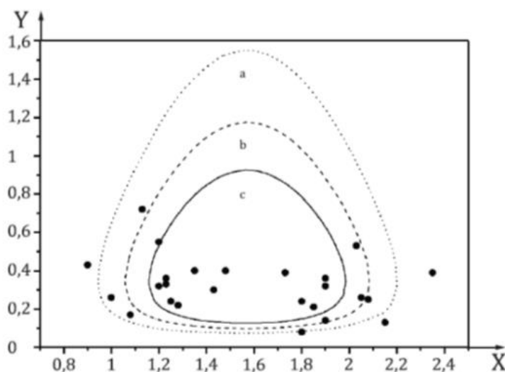
Рис.8 – График СКО и среднего значения для 25 лабораторий.
