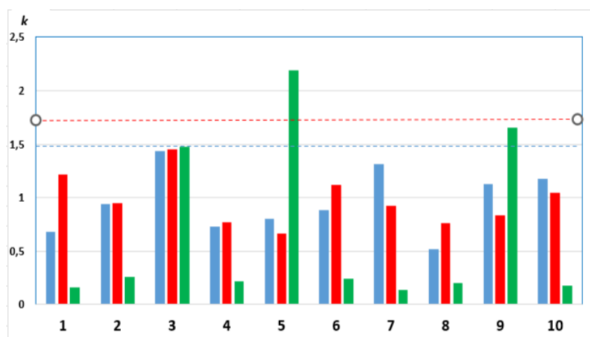
Рис. 2 – Графическое представление статистики k
