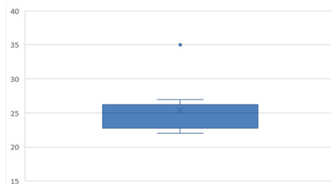
Рис.6 – Диаграмма для результатов ИЛ-1
