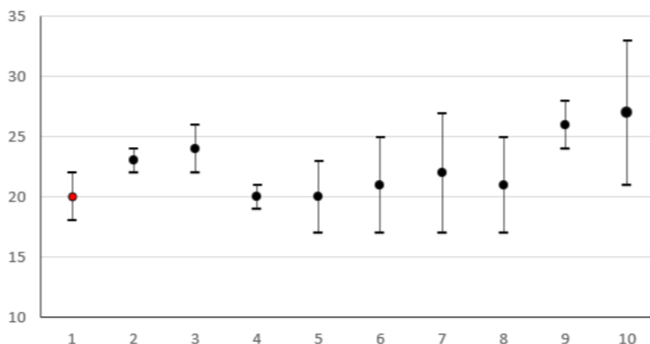
Рис. 3 – Графическое изображение результатов сличений с учетом расширенной неопределенности
