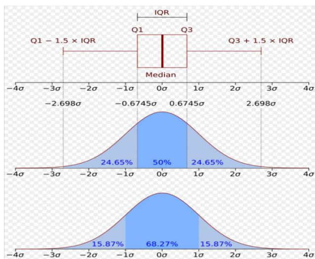
Рис. 5 – Схема соотношения диаграммы ящика с усами и нормального распределения результатов измерений
