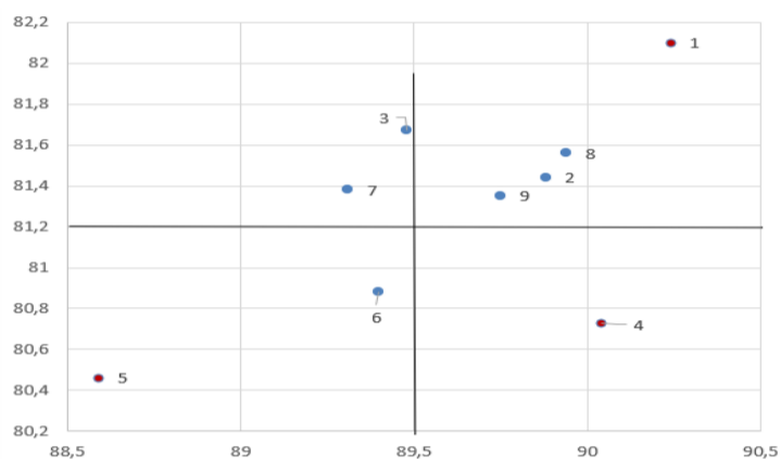
Рис. 4 – График Юдена
