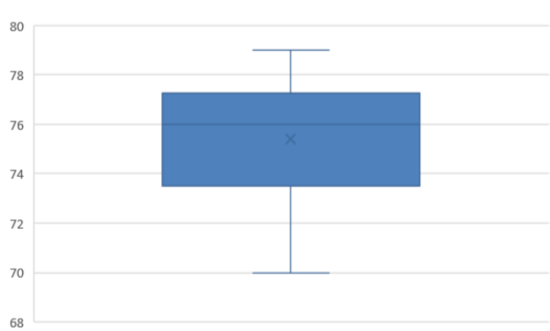
Рис.7 – Диаграмма для результатов ИЛ-2
