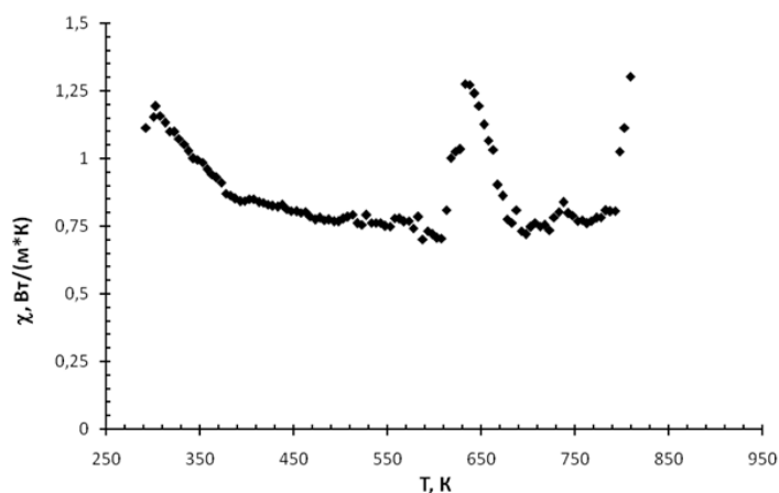
Рисунок 1 – Температурная зависимость коэффициента теплопроводности \text{Cu}_2\text{Te}
