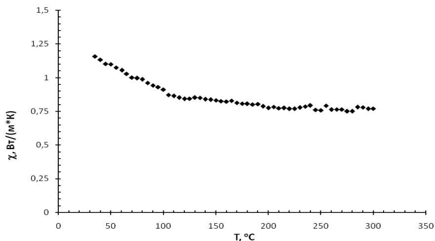
Рисунок 2 – Температурная зависимость коэффициента теплопроводности крупнокристаллического \text{Cu}_{1.97}\text{Te}
