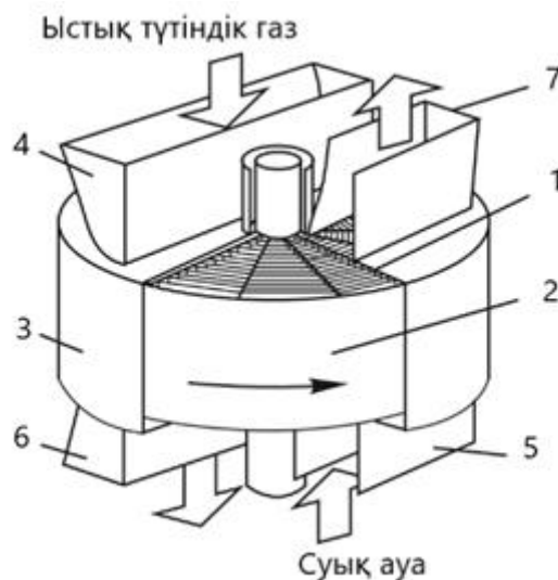
Сурет 1 - Регенеративті ауа қыздырғышының кескінді сұлбасы
