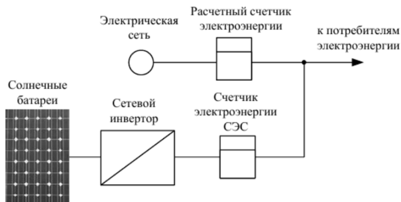
Рисунок 1 – Схема параллельно работающей с сетью солнечной электростанции
