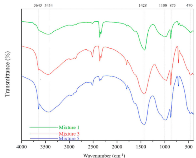
Fig. 8. FTIR-ATR analysis.
