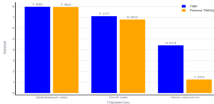
Рисунок 5 – сравнение ПВХ и резины под нагрузкой 1000 кг
