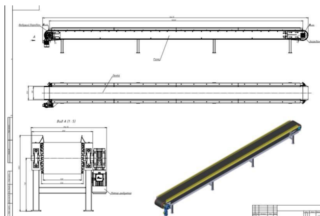
Рисунок 1 – 3D-модель ленточного конвейера
