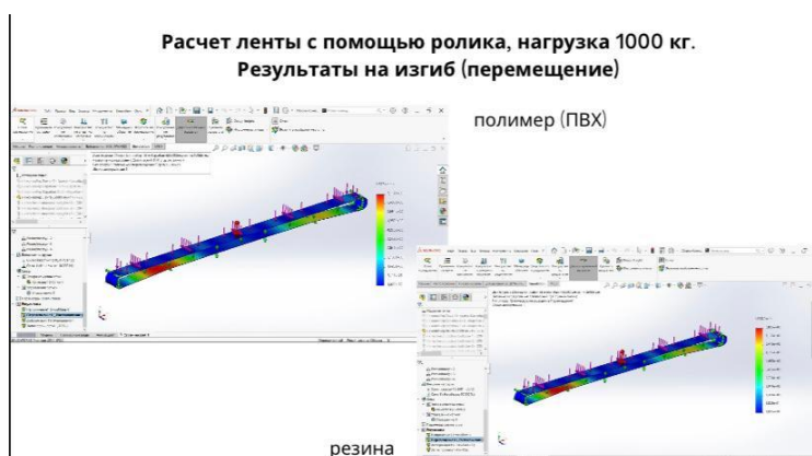
Рисунок 3 – Анализ изгиба двух материалов под нагрузкой 1000 кг
