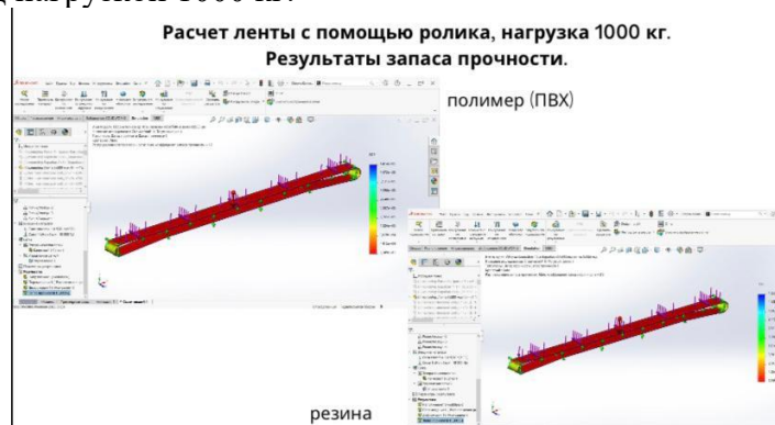
Рисунок 4 – результат прочности двух материалов под нагрузкой 1000 кг.
