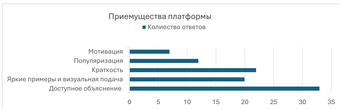
Рисунок 5 Преимущества платформы
