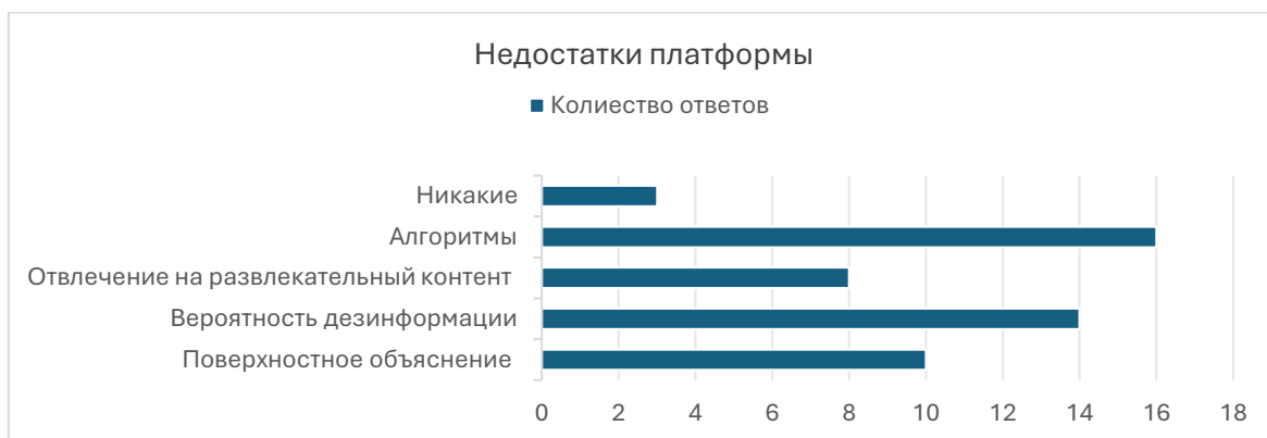
Рисунок 4 Недостатки платформы
