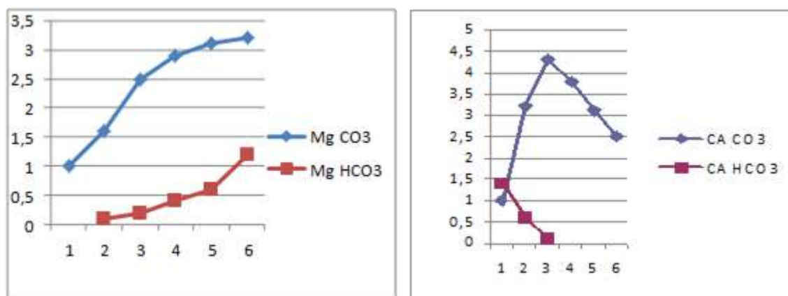
Рисунок 3,4 Зависимость содержания карбонатов и гидрокарбонатов кальция и магния от величины минерализации воды озера Балкаш (осень 2012 г.) [4]
