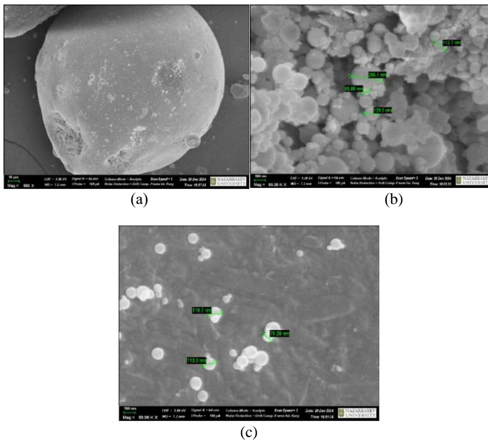
Сурет 3 Катализатордың SEM кескіндері (Cu-Al-FCC-75, (47-50-3.0) (Cu-47; Al-50; Fe-0.133; Cr- 0.627; Si- 2.205, Pх-0.015)
