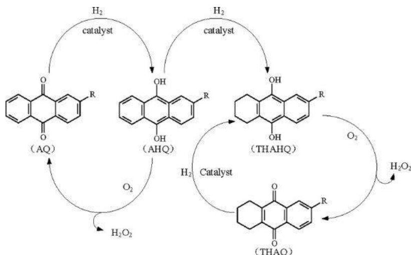
Сурет 1 Антрахинонды металл катализаторымен циклдік гидрлеу процесі
