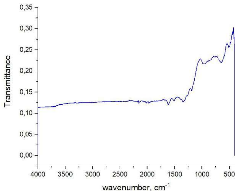
Сурет 4 Катализатордың FTIR спектрі (Cu-Al-FCC-75, (47-50-3.0)(Cu-47; Al-50; Fe-0.133; Cr- 0.627; Si- 2.205, Pх-0.015)
