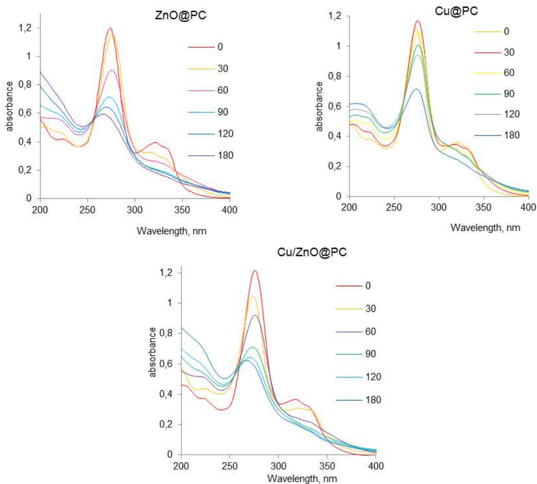
Сурет 1 Композиттік мембраналардың ZnO@PC (а), Cu@PC (b) және Cu/ZnO@PC (c) қатысуымен УФ-көрінетін жарық әсерінен NOR ыдырау кезіндегі жұтылу спектрлері (NOR концентрациясы – 10 мг/л, температура – 30 °С, каталитикалық мембрана өлшемі – 2×2 см).
