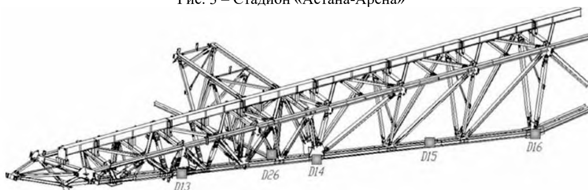
Рис. 4 - Схема установки акустико-эмиссионных датчиков на несущие конструкции покрытия крытого стадиона «Астана-Арена»
