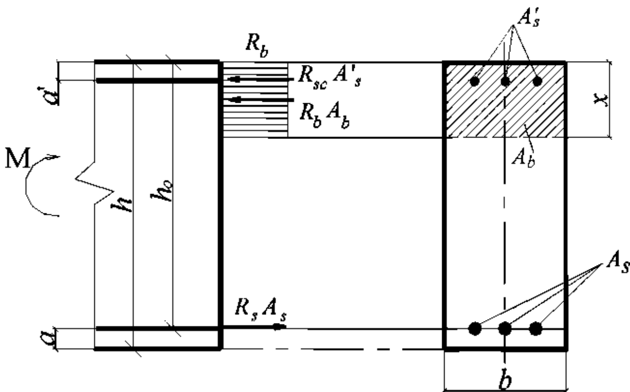
Сурет 1 – Күш схемасы және кернеулер эпюрасы бойынша есептелетін центрден тыс сығылған бетон элементтерінің бойлық осіне қалыпты қимада созылған аймақ бетонының кедергісін есепке алмағандағы беріктігі
