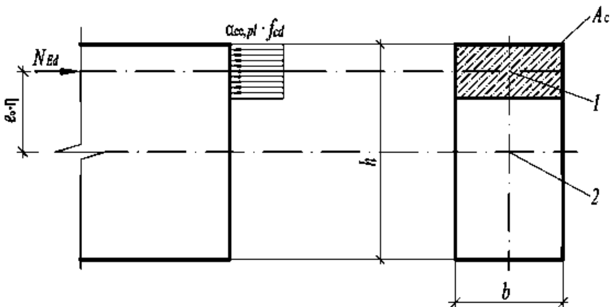
Сурет 2 – Бетонның созылған аймағының кедергісін есепке алмағанда беріктігі бойынша есептелетін орталықтан тыс сығылған бетон элементінің бойлық осіне қалыпты қимадағы күш схемасы мен кернеулер эпюрасы (1-сығылған аймақ ауданының A_c ауырлық центрі, 2- бүкіл қиманың ауданы)
