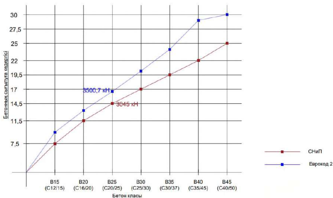
Сурет 3 – СНИП және Еурокод 2 есептеу әдістері бойынша бағанның жүк көтергіштік қабілеті
