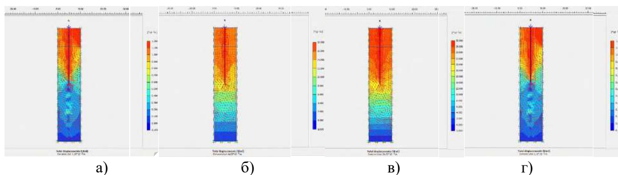
Сурет 2. Қадаға әртүрлі жүктемелер кезіндегі ығысу түрлері: а - 360 кН жүктеме; б - 720 кН жүктеме; в - 1200 кН жүктеме; г - түсіруден кейінгі қалдық жылжулар
