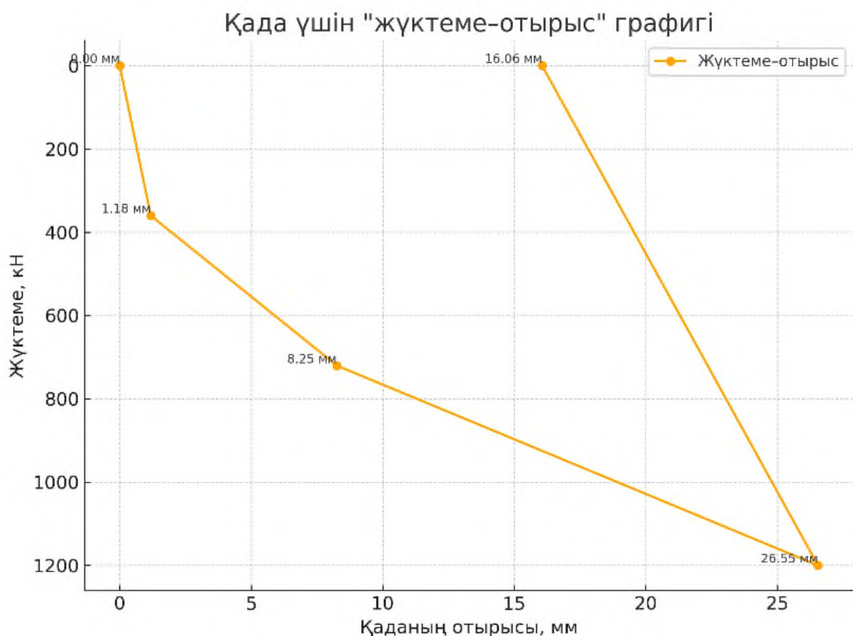
Сурет 6 - Қада отырысы графигі
