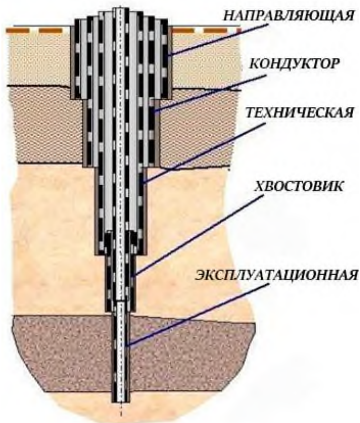
Сурет 1. Ұңғыма конструкциясы
