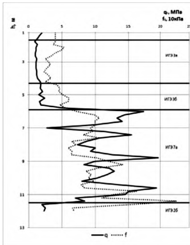
Рисунок 2 – Автоколебания сопротивления погружению зонда ( q_c )
