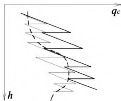
Рисунок 1 – Сравнение сопротивления погружению зонда при различных системах регистрации
