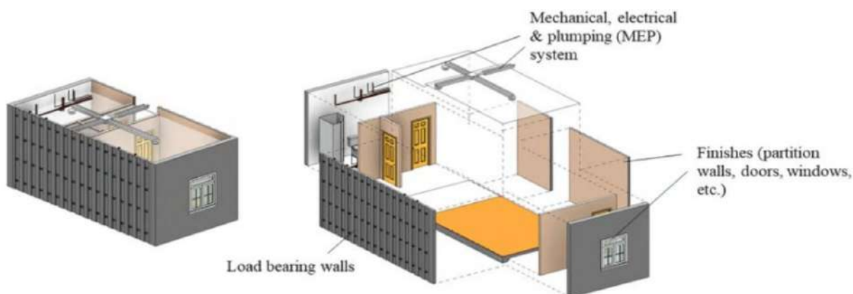
Рисунок.1 – Несущая модульная система
