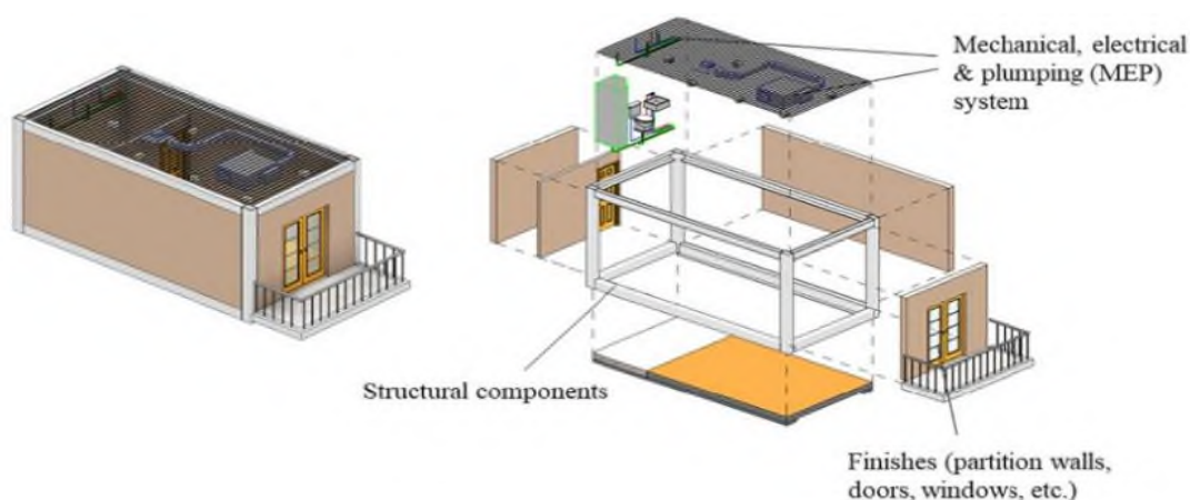
Рисунок.2 – Каркасная модульная система
