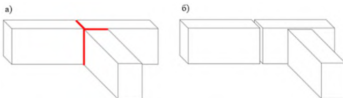
Рис. 4 Перевязка стены из фундаментных блоков: а) фактическое состояние на момент обследования с открытым вертикальным швом, способствующим проникновению воды в узле 1/Б, б) решение узла примыкания фундаментных блоков, препятствующее проникновению воды (без вертикального шва в узле по осям 1/Б)
