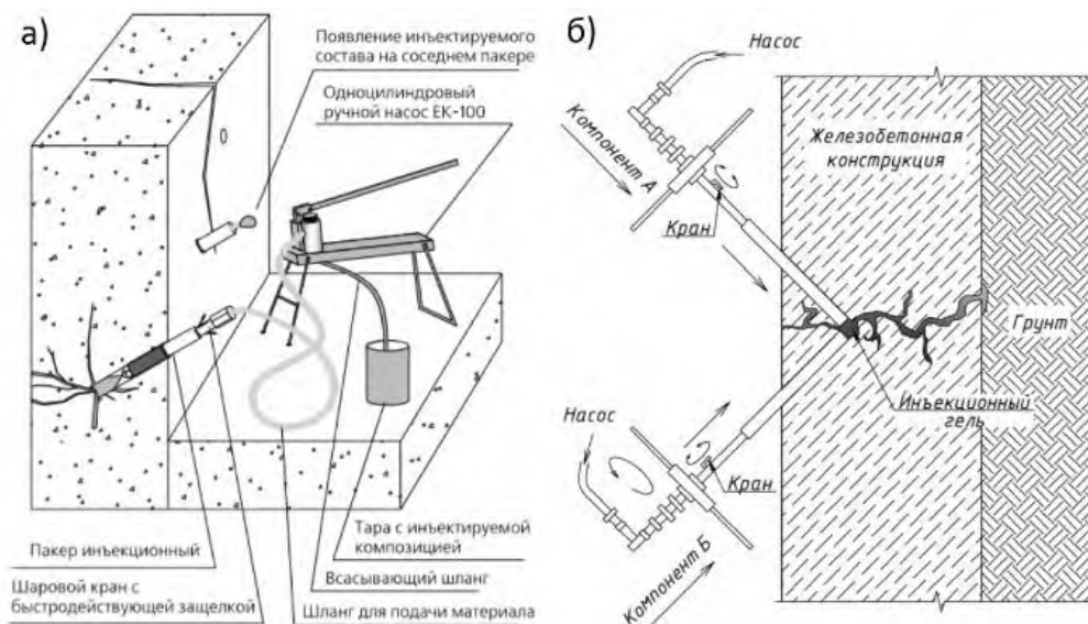
Рис. 7 Технологический процесс(а) и схема(б) инъектирования трещин железобетонных конструкций
