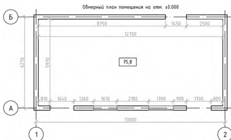
Рис. 2 Обмерный план нежилого помещения в ЖК «BASKAR U-4» (первый этаж, угловая)
